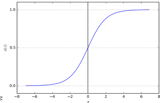
Sigmoid
